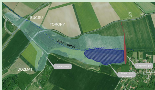
Dozmati árvízcsúcs-csökkentő tározó helyszínrajza
